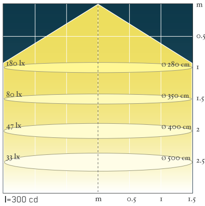
fluorescent, PAR 38 - E27, 20W, 110°
