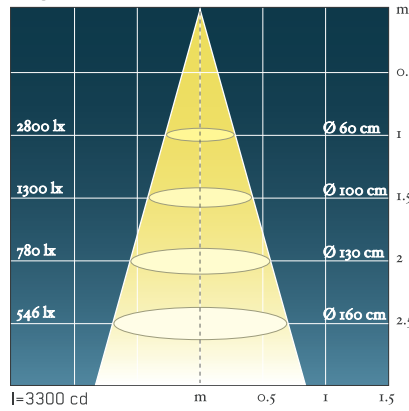
halogen reflector, PAR 30 - E27, 100W, 30°
